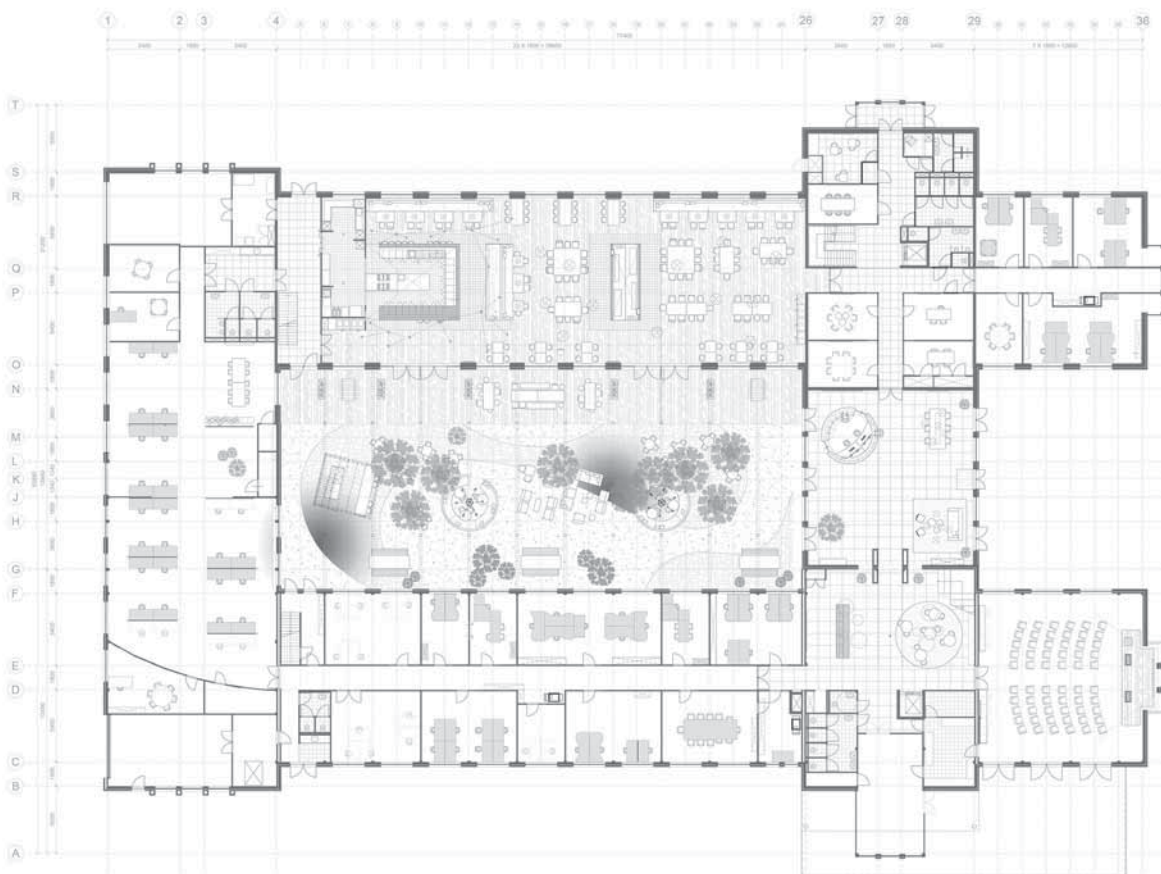
PLATTEGROND Begane grond.
